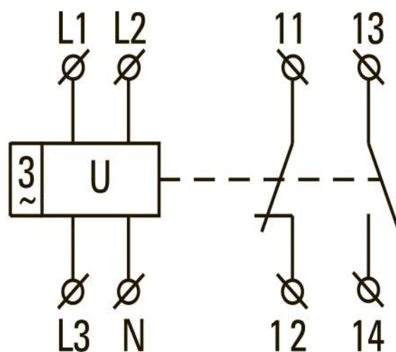
Рис. 4 Электрическая схема
