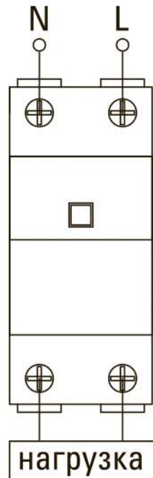
Рис. 1 Схема подключения реле напряжения RVb
