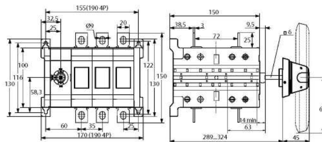
Ревёрсивный рубильник 315-400 А
