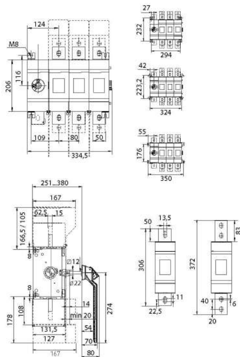
Рубильник 1000-1600 А
