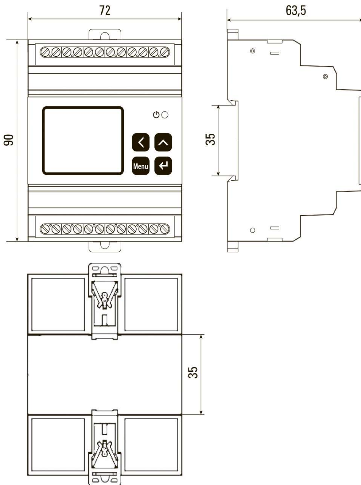
Рис. 1 Форма и размеры счетчика (мм)
