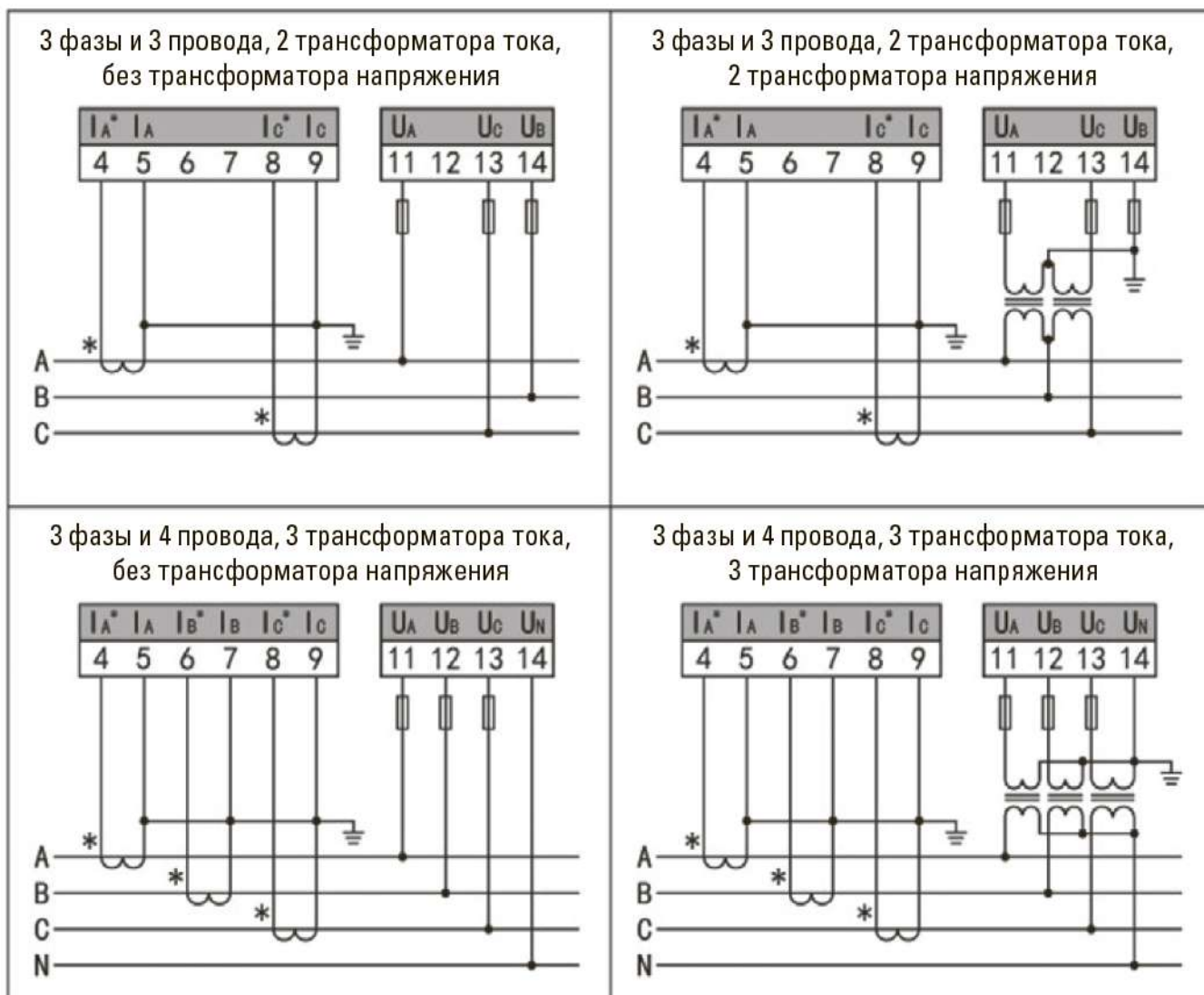
Рис. 2 Схема подключения
