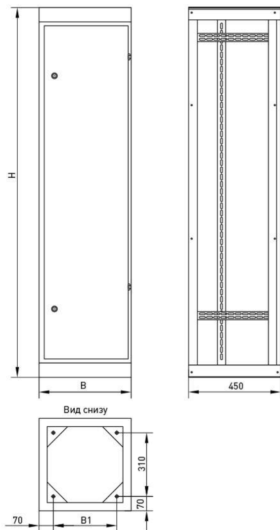
ВРУ-1 IP 31
