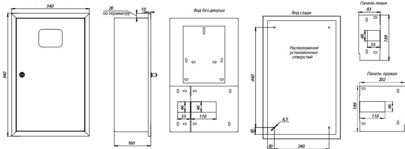
ЩУРВ-3/9, ЩУРВ-3/12
