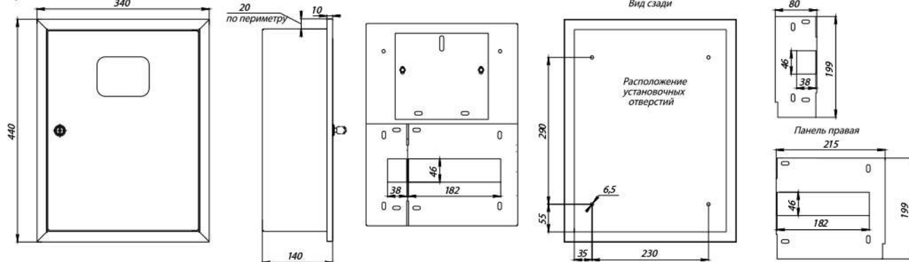
ЩУРВ-3/9, ЩУРВ-3/12
