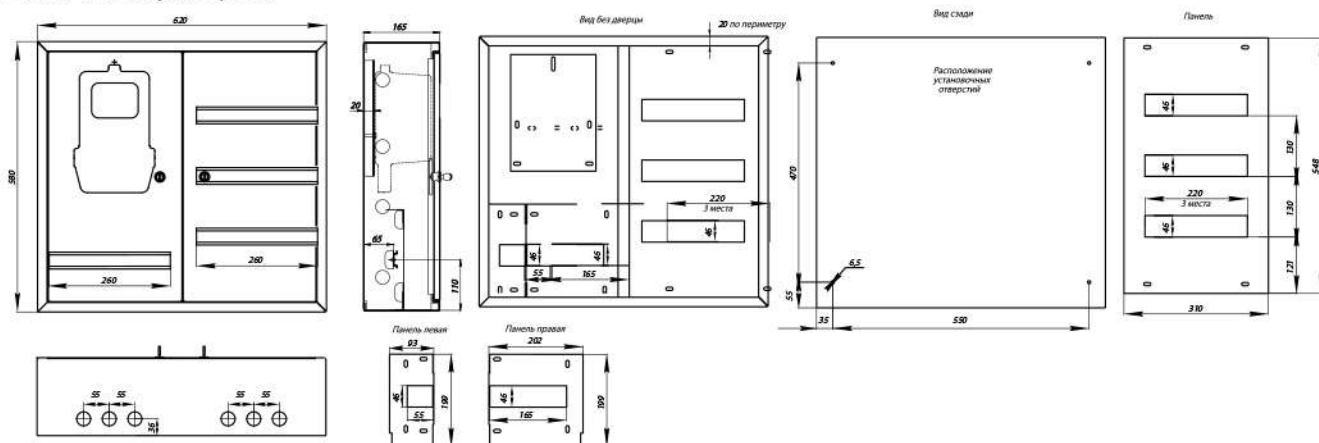
ЩУРН-3/48 однодверный
