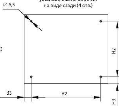
Рис. 1. Расположение установочных отверстий на виде сзади (4 отв.)
