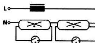
Рис. 2. Схемы электрические компенсированные
