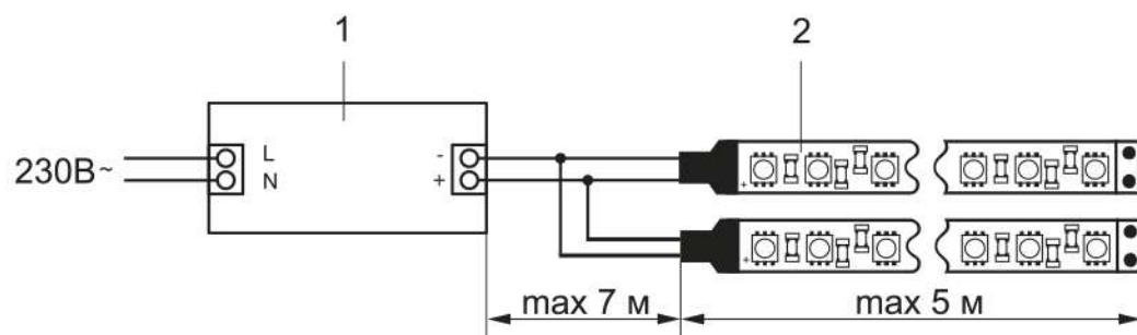
Рисунок 3 – Схема подключения одноцветной светодиодной ленты
