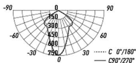
PSP-S 212 2x8W
