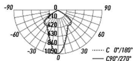
PSP-S 213 3x8W
