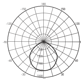
PFL-S2 70w 6500K IP65
