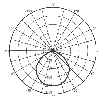
PFL-S2 70w 6500K IP65
