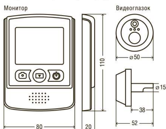
Рисунок 1. Габаритные размеры, мм
