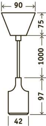
Габаритные размеры
