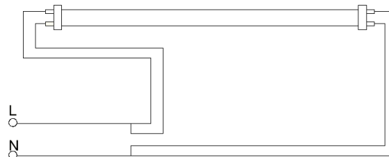
Схема подключения LB213
