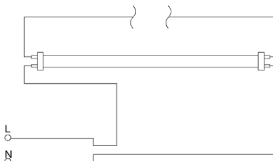
Схема подключения LB213
