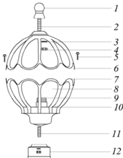
1 – балясина; 2 – резьбовое крепление; 3 – пружина; 4 – гайка; 5 – винты; 6 – верхняя крышка; 7 – нижняя крышка; 8 – рассеиватель; 9 – патрон; 10 – ламподдержатель; 11 – резьбовое крепление; 12 – основание.
