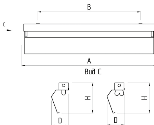
Светильники с отражателями под лампы T5 (G5), T8 (G13)
