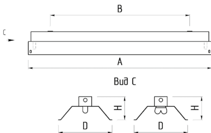
Светильники с отражателями под лампы T5 (G5), T8 (G13)
