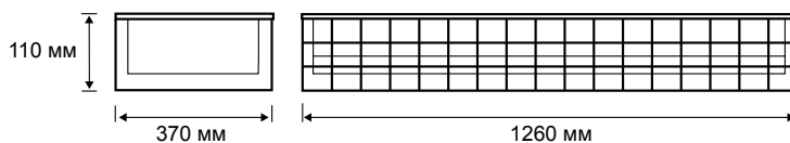
Защитная решетка
