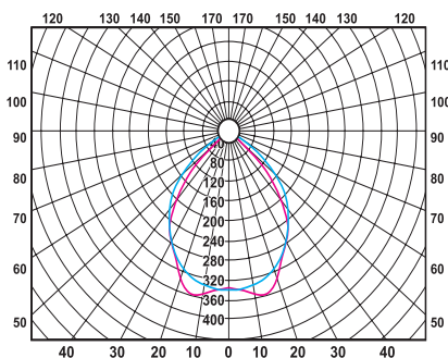
Кривая светораспределения - П Тип кривой силы света - Г КПД - 56%
