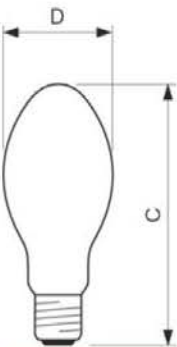
HPI Plus 400W/645 BU E40
