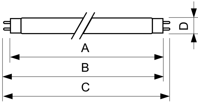
TL-D 36W/54-765
