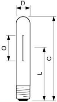
SON-T 250W E E40
