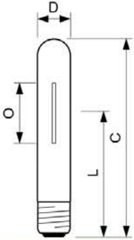
SON-T 150W E E40
