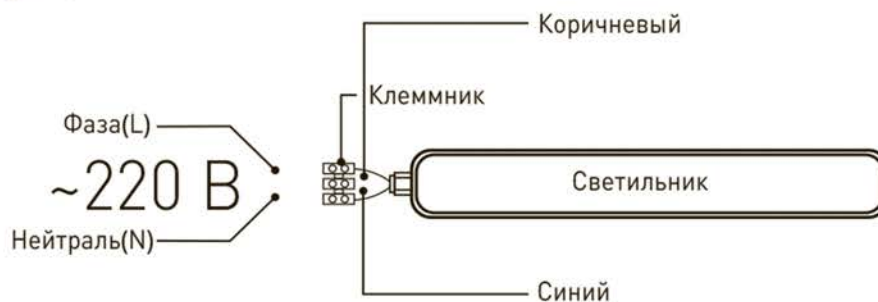
Рис.1. Схема подключения светильника к сети 220В.
