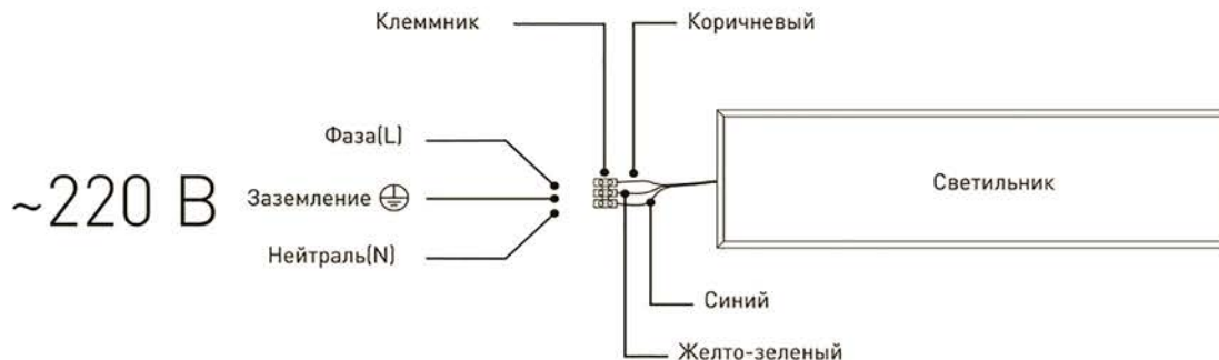
Рис.1. Схема подключения светильника к сети 220В.
