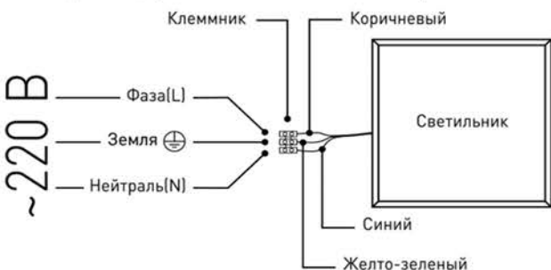
Рис.1. Схема подключения светильника SPO-6-48 к сети 220В.
