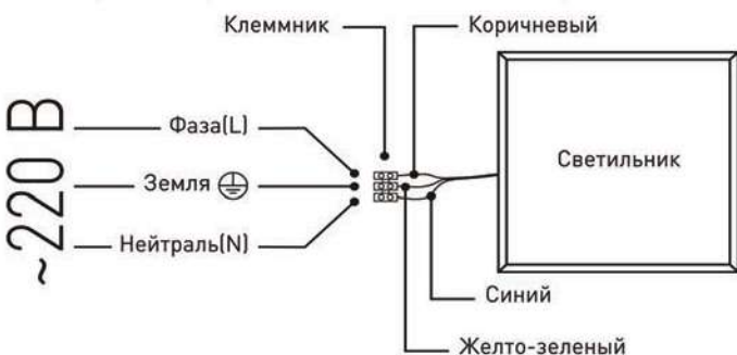
Рис.1. Схема подключения светильника SPO-6-48 к сети 220В.
