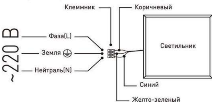
Рис.1. Схема подключения светильника SPO-6-48 к сети 220В.
