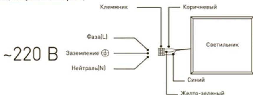
Рис.1. Схема подключения светильника к сети 220В.
