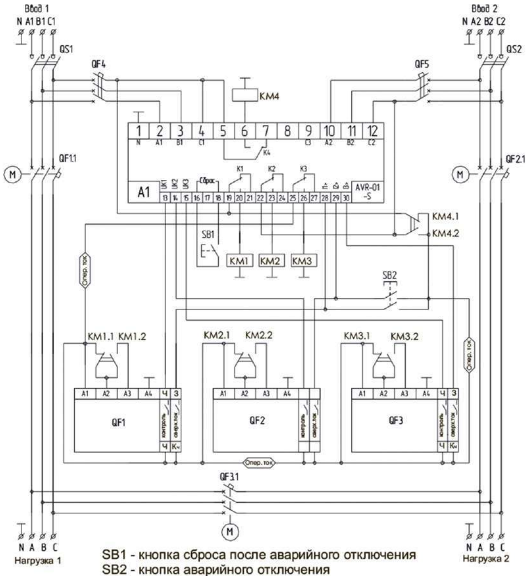
Схема подключения AVR-01-S с моторприводами (на примере ВА57-35)
