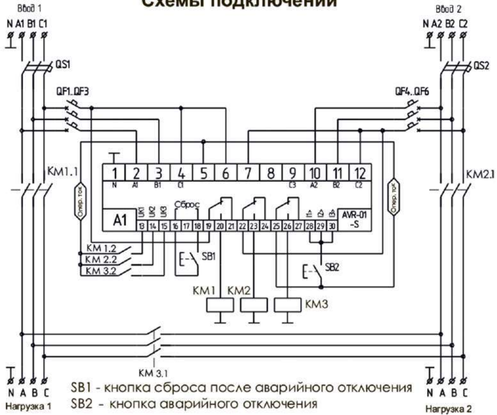
Схема подключения AVR-01-S с контакторами.
