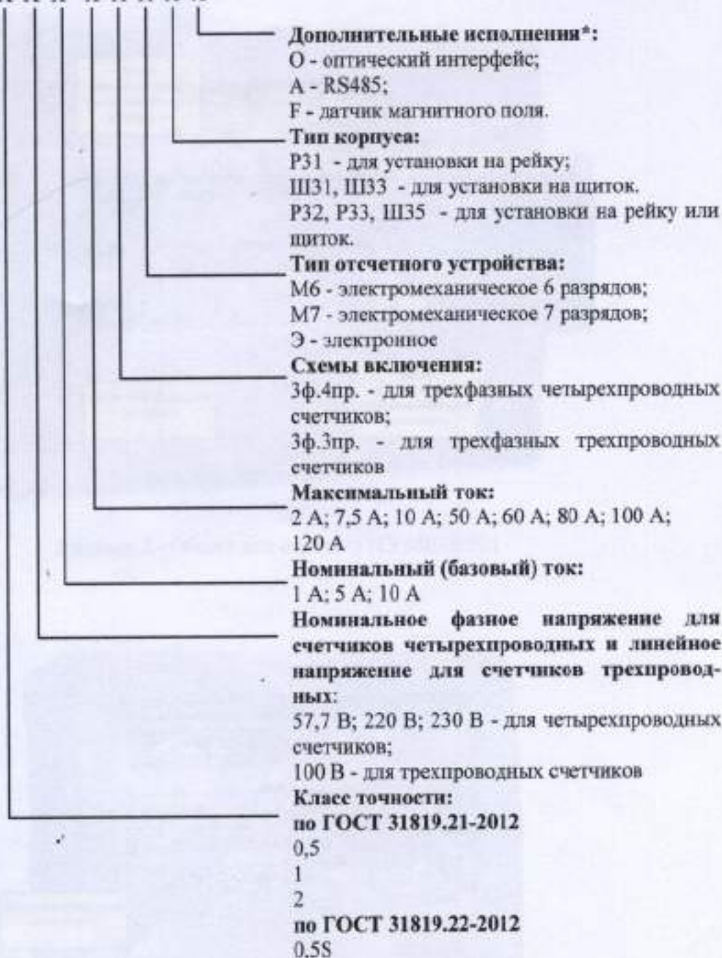
Рисунок 1 - Структура условного обозначения счетчиков
