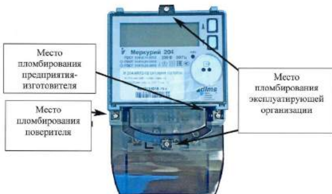
Рисунок 1 – Общий вид счетчиков модификаций «Mercury 204» и «Mercury 204» с указанием мест пломбирования и нанесения знака поверки
