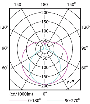
LEDtube 1200mm 16W 740 T8 CN I G
