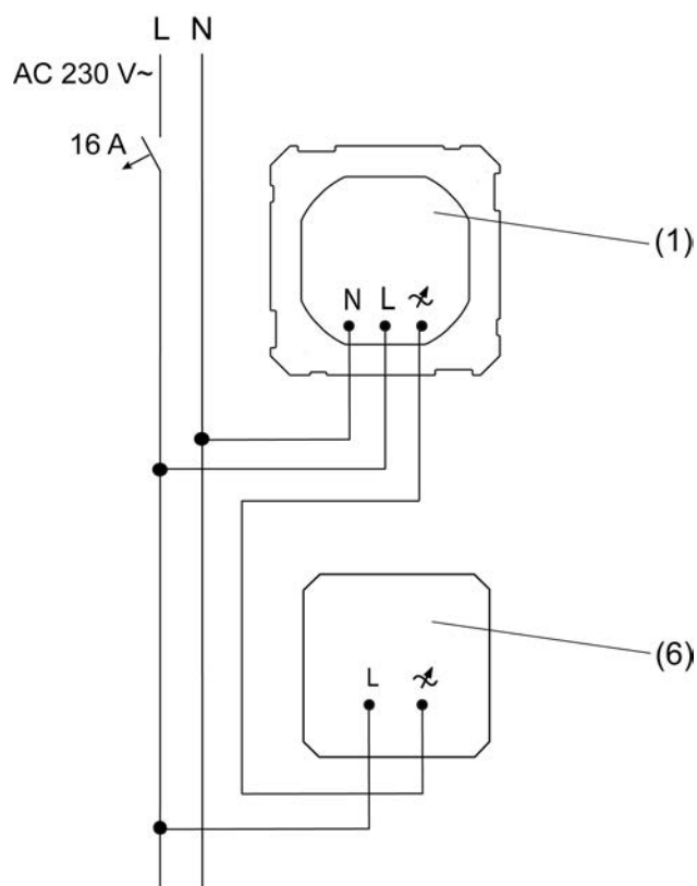
рисунки 2: Для осветительных насадок с регулированием яркости: схема подключения для двухпроводного светодиодного регулятора яркости (6)
