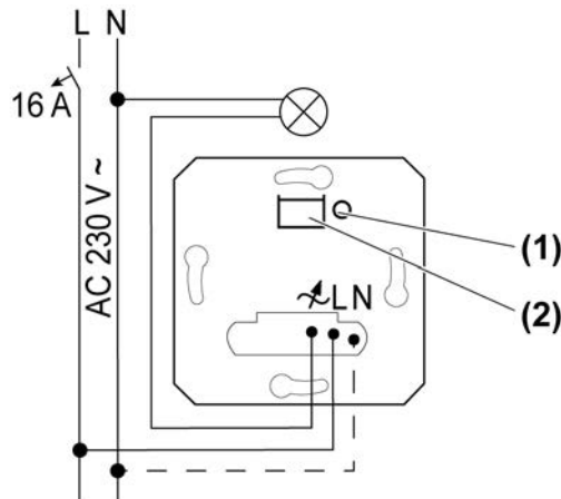
рисунок 1: Монтажная схема
