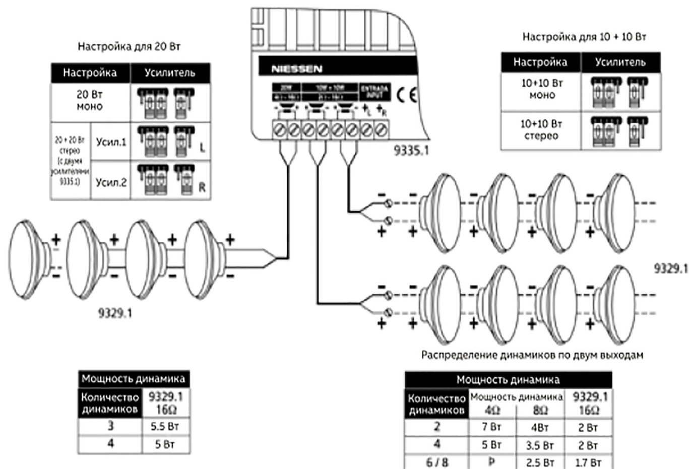
Схема подключения динамиков 9329.1 к усилителю звука 9335.1
