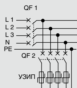
Трехфазная система
