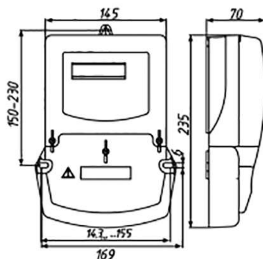
Рисунок А.2 — Тип корпуса Ш33
