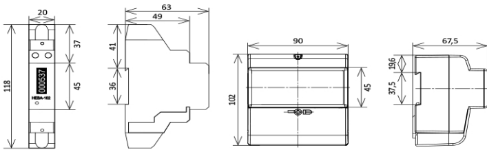
Внешний вид счетчиков НЕВА 102 и НЕВА 105
