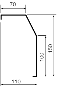
Габаритные размеры
