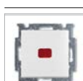
Выключатель с клавишей 1)2) переключатель с N-клеммой с лампой подсветки Номинальное напряжение: 250 В перем. тока Номинальный ток: 10 АХ IEC 60669-1
