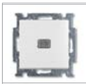
Выключатель без фиксации с клавишей и нейтральным символом 1) 1 полюс, нормально-открытый контакт с N-клеммой Номинальное напряжение: 250 В перем. тока Номинальный ток: 10 А IEC 60669-1
