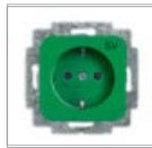
Механизм розетки SCHUKO® с маркировкой с безвинтовыми клеммами 2 P + E цветная маркировка центральной платы и цоколя Номинальное напряжение: 250 В перем. тока Номинальный ток: 16 А
