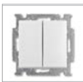
Выключатель с клавишей 2-х клавишный Номинальное напряжение: 250 В перем. тока Номинальный ток: 10 АХ IEC 60669-1
