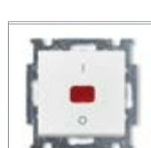
Выключатель с клавишей для 2-полюсных контрольных выключателей с лампой подсветки Номинальное напряжение: 250 В перем. тока Номинальный ток: 20 АХ IEC 60669-1
