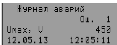
Рисунок 5.17 – Индикатор в состоянии Просмотр журнала аварий
