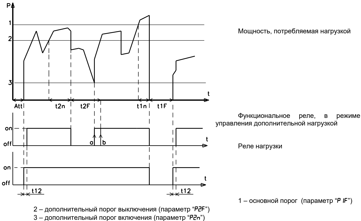
Рисунок 1.3 - Работа OM-310 в режиме ограничения мощности при r2r=2
