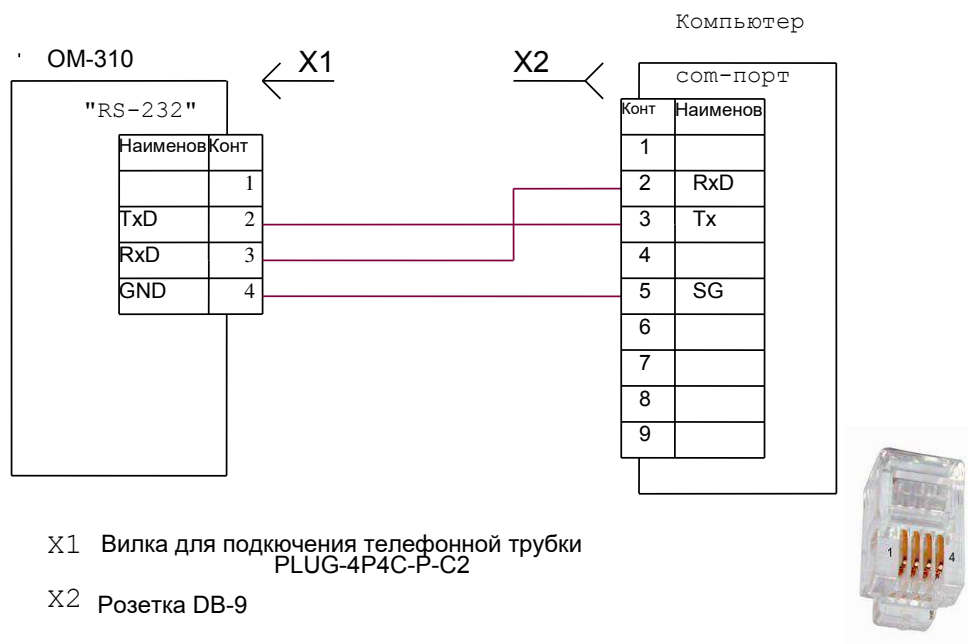
Рисунок 2.2 - Схема подключения ОМ-310 к компьютеру
