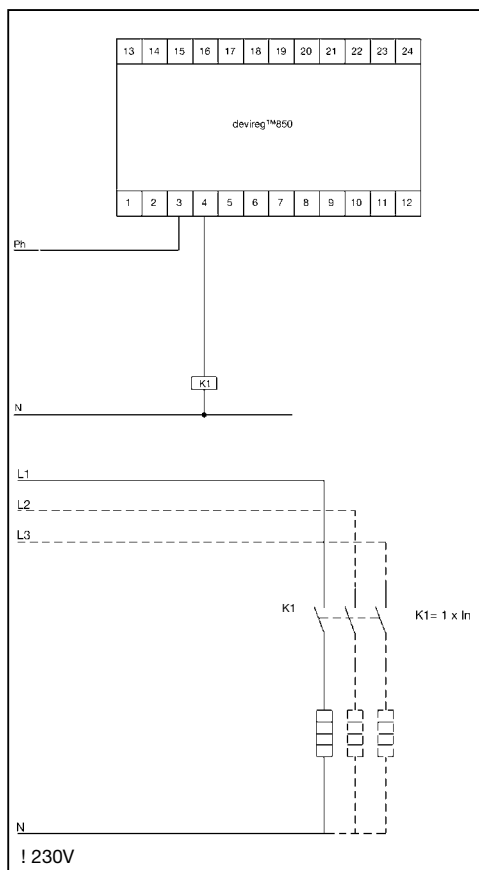
Рис. D. Кровля, 1-3 фазы, 1-3 кабеля на 230
