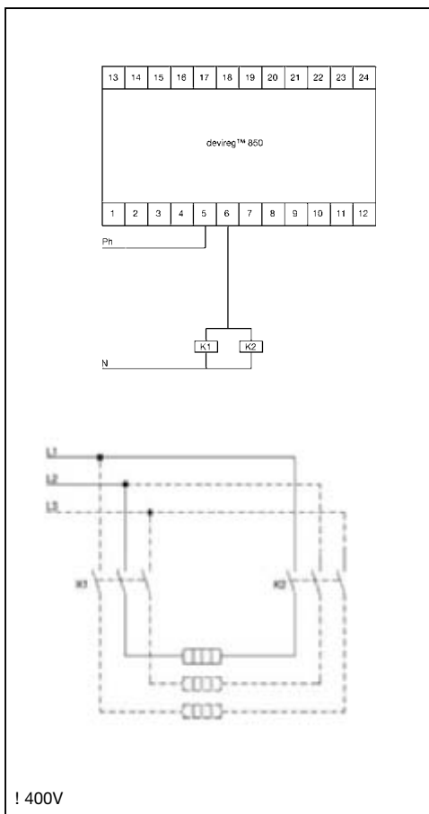
Рис.Г. Грунт, прямое подключение кабеля
