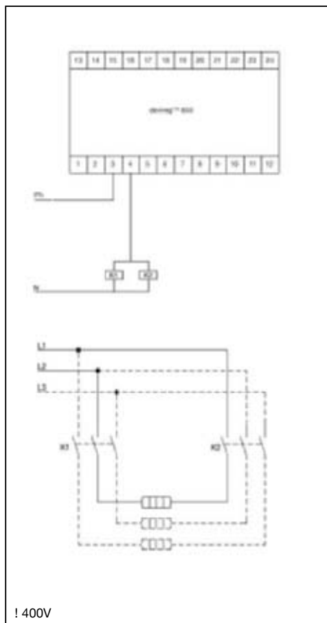
Рис.Н. Кровля, прямое подключение кабеля
