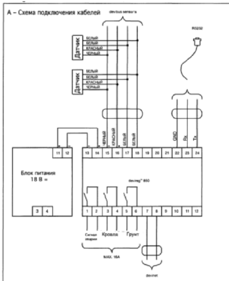
Рис. А. Общая схема подключения с источником питания =18В (см. Приложение А)
