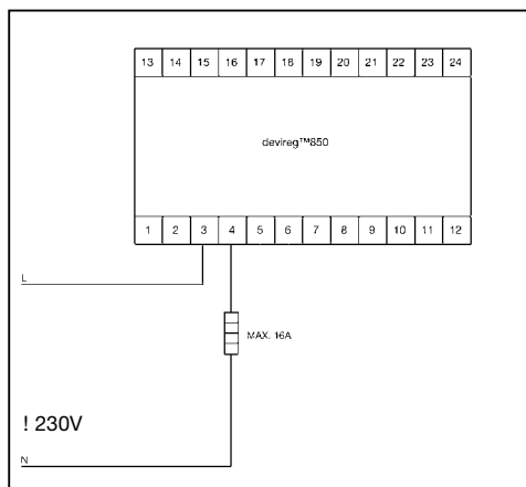
Рис.Н. Кровля, прямое подключение кабеля
