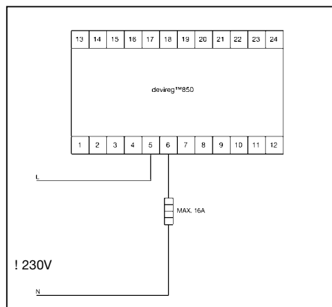
Рис.Г. Грунт, прямое подключение кабеля
