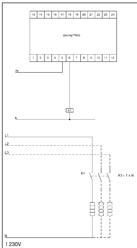
Рис. С. Грунт, 1-3 фазы, 1-3 кабеля на 230В
