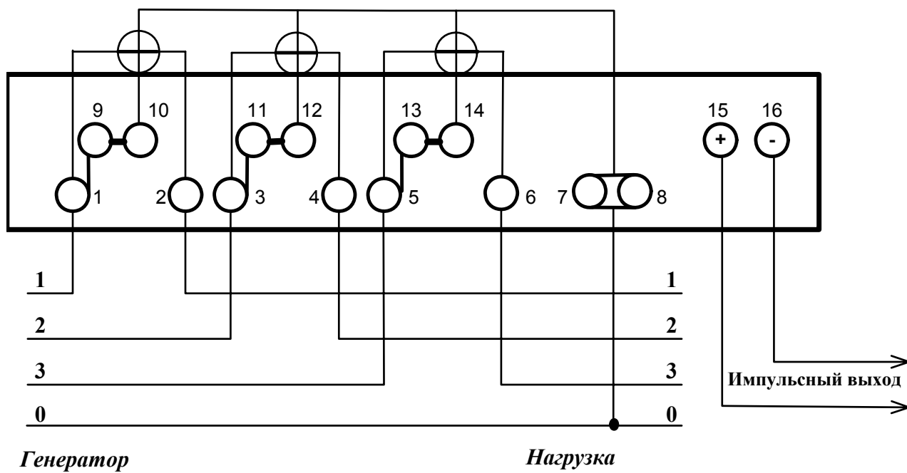
Рисунок Б.1 – Схема непосредственного подключения счётчика
