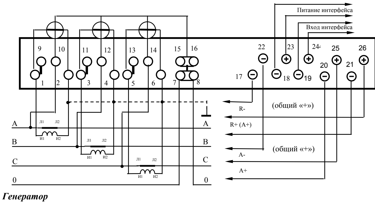
Рисунок I.2 - Схема подключения счётчика с помощью трёх трансформаторов тока.
