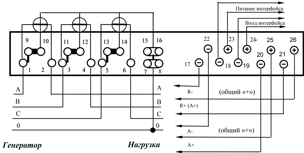
Рисунок I.1 - Схема непосредственного подключения счётчика.
