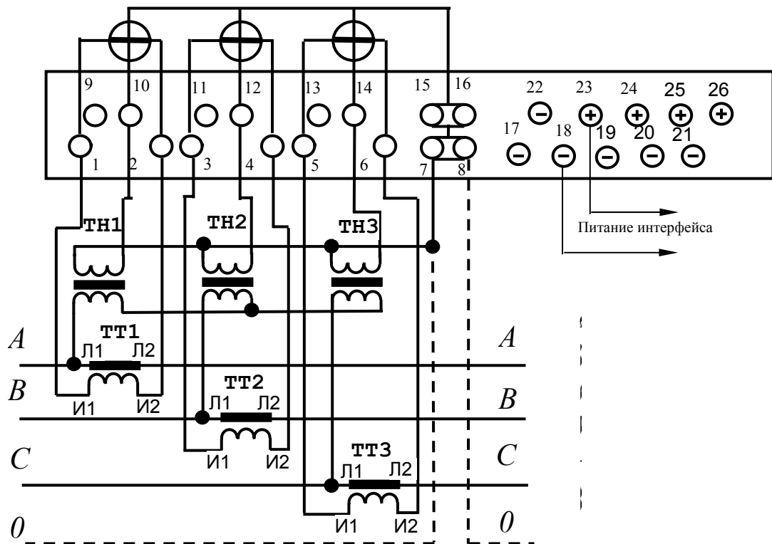
Рисунок II.1 - Схема подключения счётчика к трёхфазной 3- или 4-проводной сети с помощью трёх трансформаторов напряжения и трёх трансформаторов тока.
