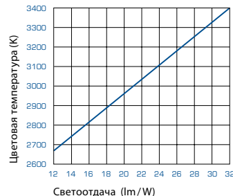
Взаимосвязь между светотдачей и цветовой температурой
