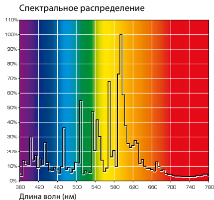
Рис. 6: Спектр газоразрядной лампы цвета „ww“ (белый теплый): смешение разных цветов образует белый цвет освещения с хорошей цветопередачей.
